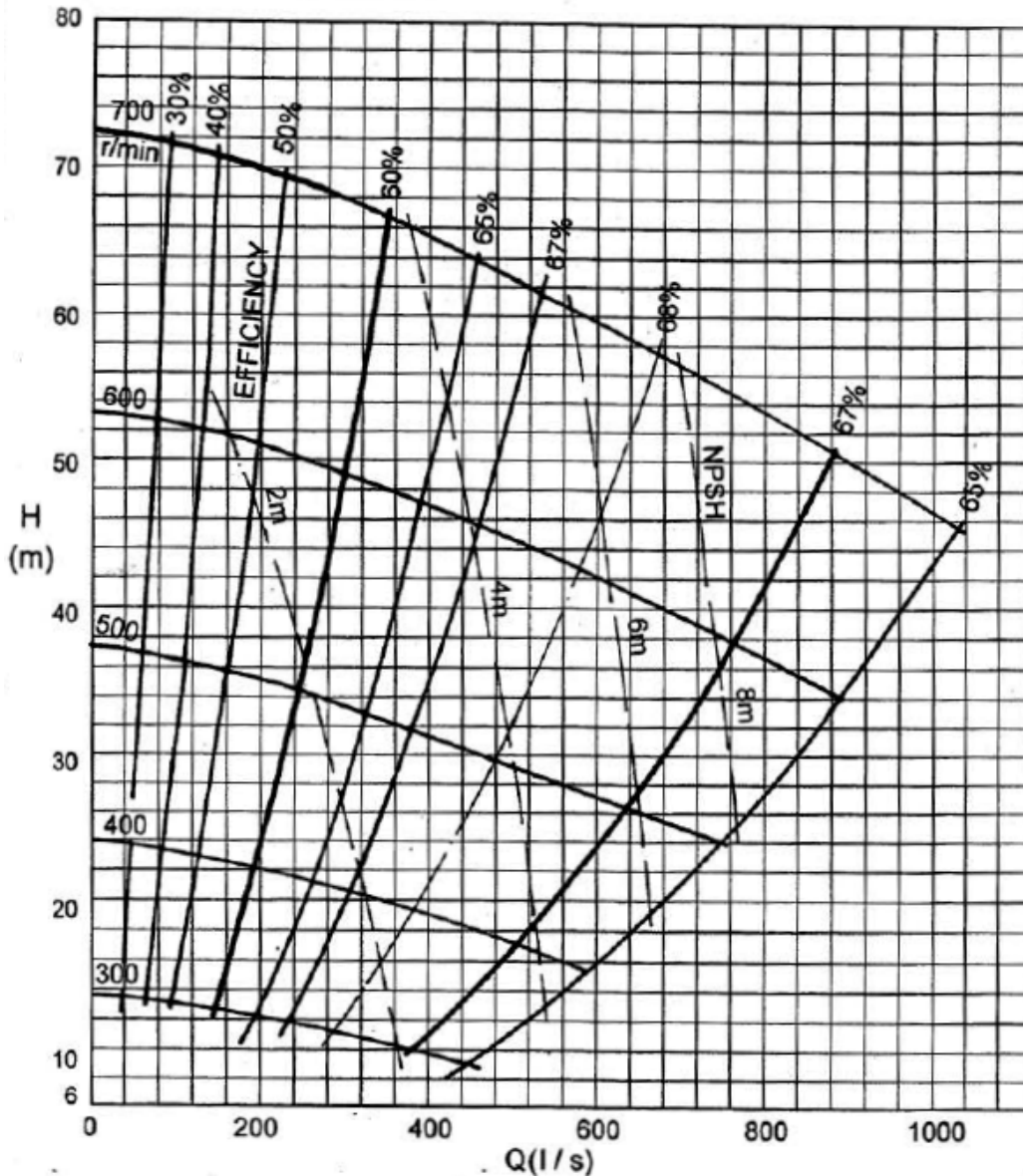
Характеристики насоса DRW 14/12G-G (Гравий, песок)
