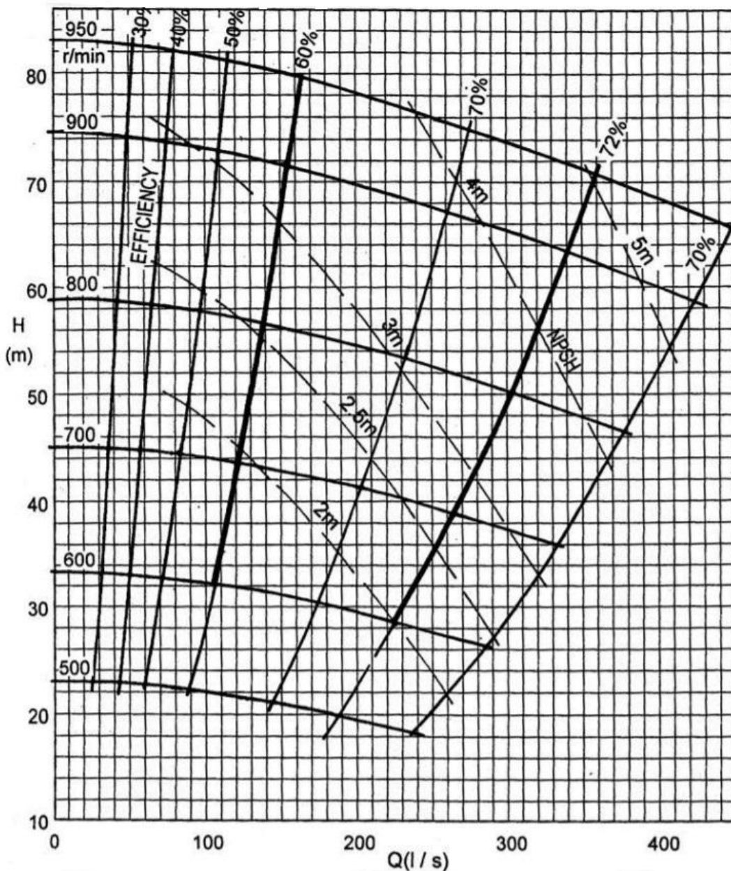
Характеристики насоса DRW 10/8S-G (Гравий, песок)
